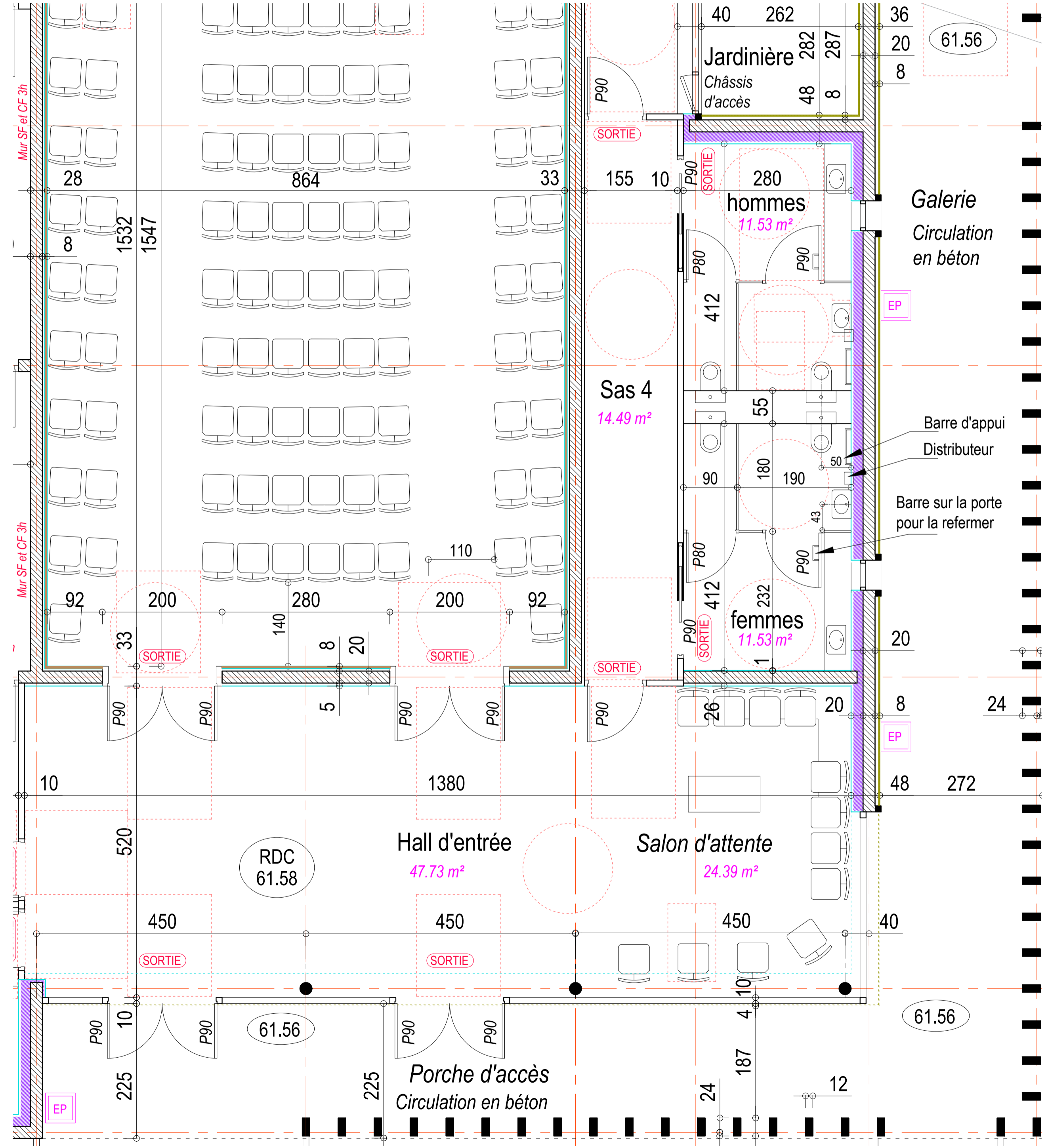
Plan des sanitaires accessibles PMR
