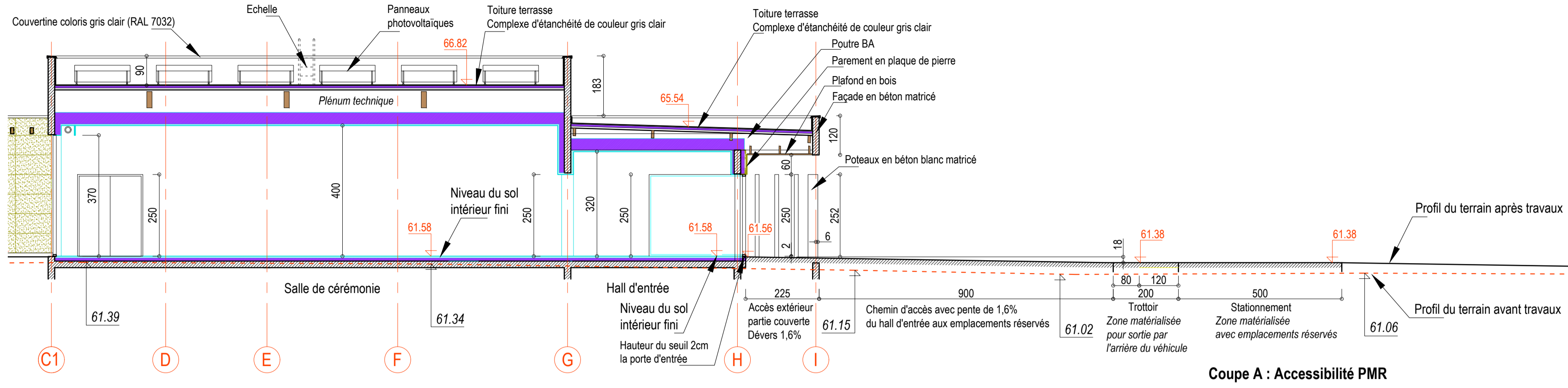
Coupe A : Accessibilité PMR
